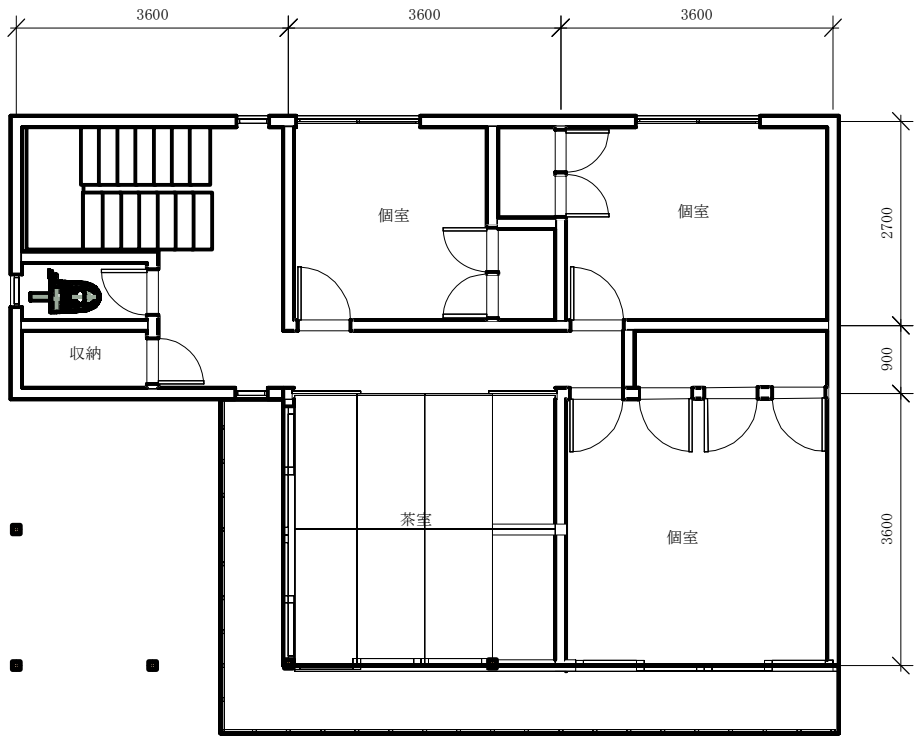
2階平面図
