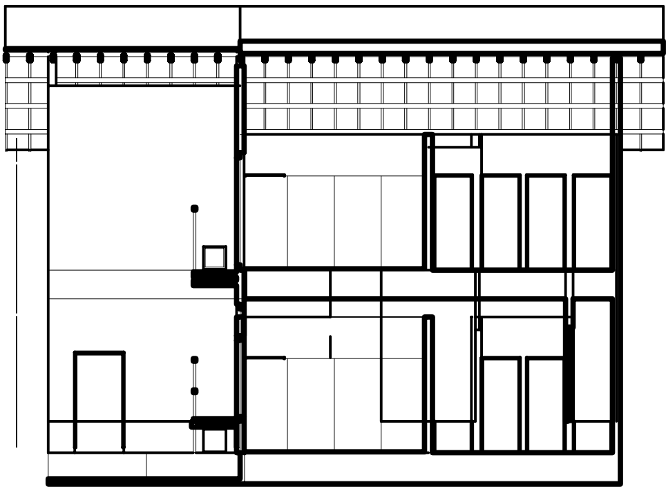
断面図 1:100
