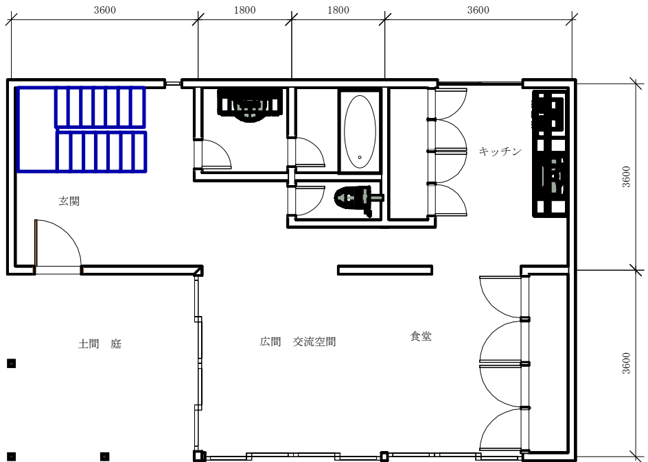
1階平面図 1:100
